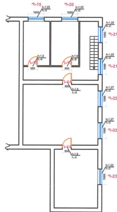
ՄԻՋՆԱՅԱՐԿԻ ՀԱՏԱԿԱԳԻԾ 2,800 ՆԻՇԻ ԿՐԱ
